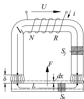
Slika 3.26 Skica elektromagneta
