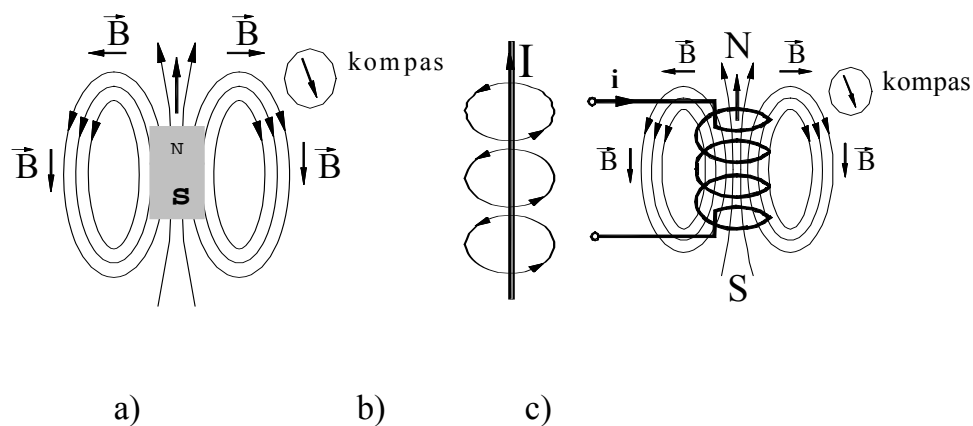
Slika 3.1 Dvodimenzionalni prikaz magnetnog polja; a) Stalnog magneta, b) Ravnog provodnika, c) Solenoida
