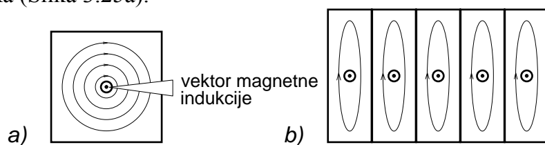
Slika 3.25 Vrtložne struje u; a) Punom magnetnom kolu i b) Magnetnom kolu sačinjenom od limova.
